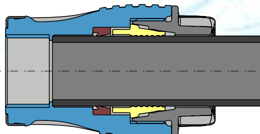
Låst tryckmutter
