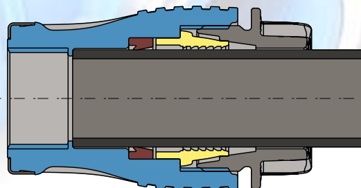
Öppen tryckmutter
