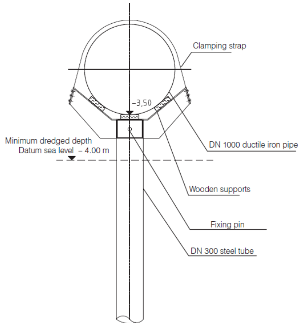
Fig. 5.9 Djup fundament (förankring) för en DN 1000 segjärnsledning
