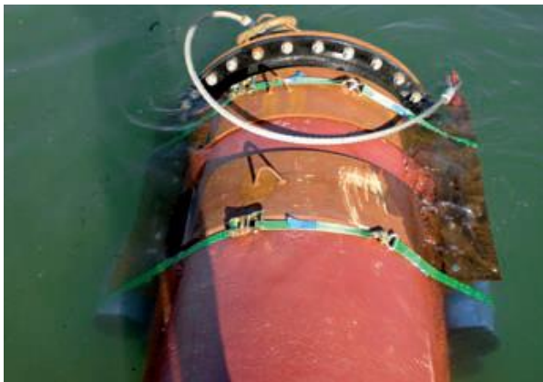
Fig. 5.1 Draghuvud med flytkroppar (PE-rör)
